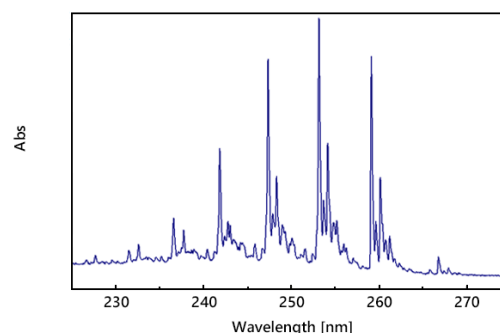
Benzene spectrum
